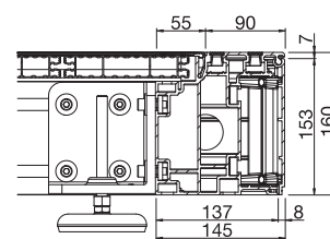
SB4700 Querschnitt
