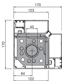
Schnitt Fussplatte/Eckstützenprofil
